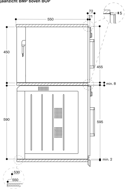
Zijaanzicht BMP boven BOP
