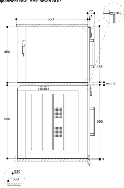
Zijaanzicht BSP, BMP boven BOP
