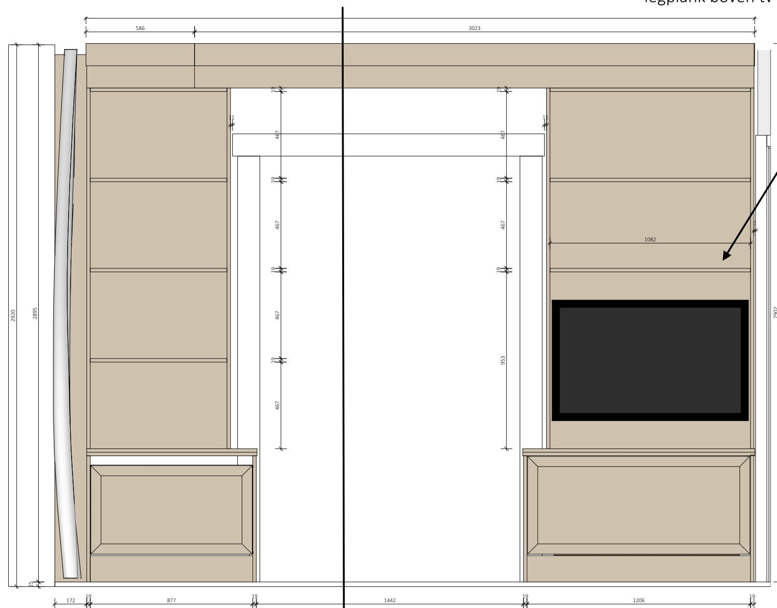
zijaanzicht A
